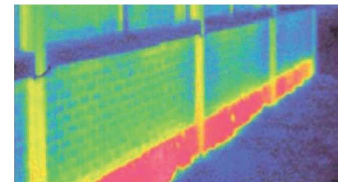
Przykład mostka termicznego u podnóża ściany
